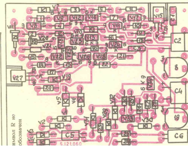
УЗЕЛ 4 (А4)
