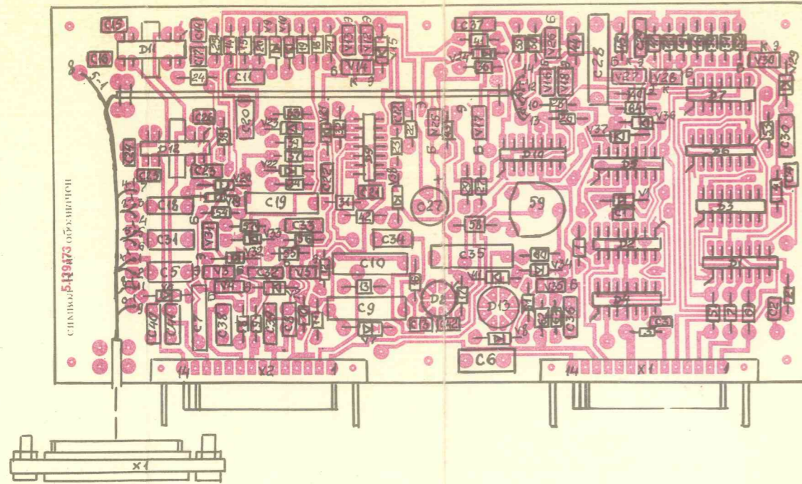
УЗЕЛ 2 (А2)
