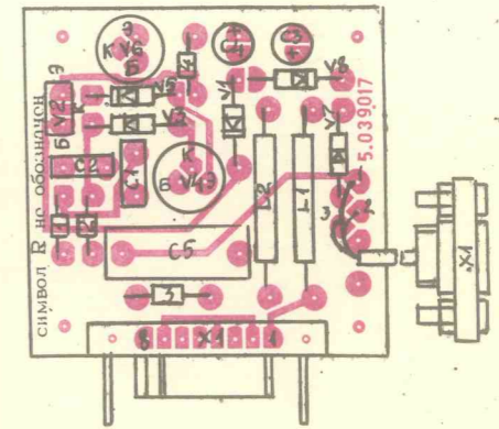
УЗЕЛ 5 (А5)
