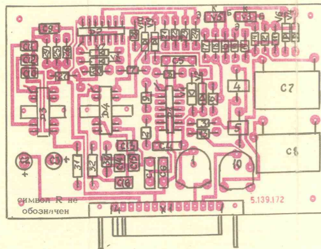
УЗЕЛ 3 (А3)
