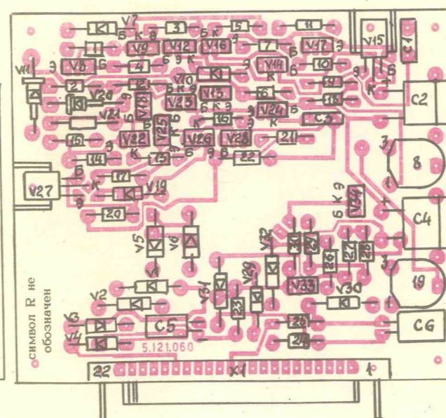
УЗЕЛ 4 (А4)
