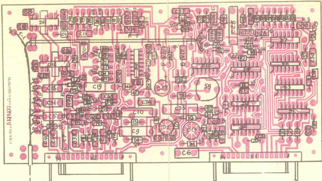
УЗЕЛ 2 (А2)
