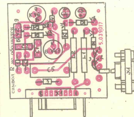
УЗЕЛ 5 (А5)
